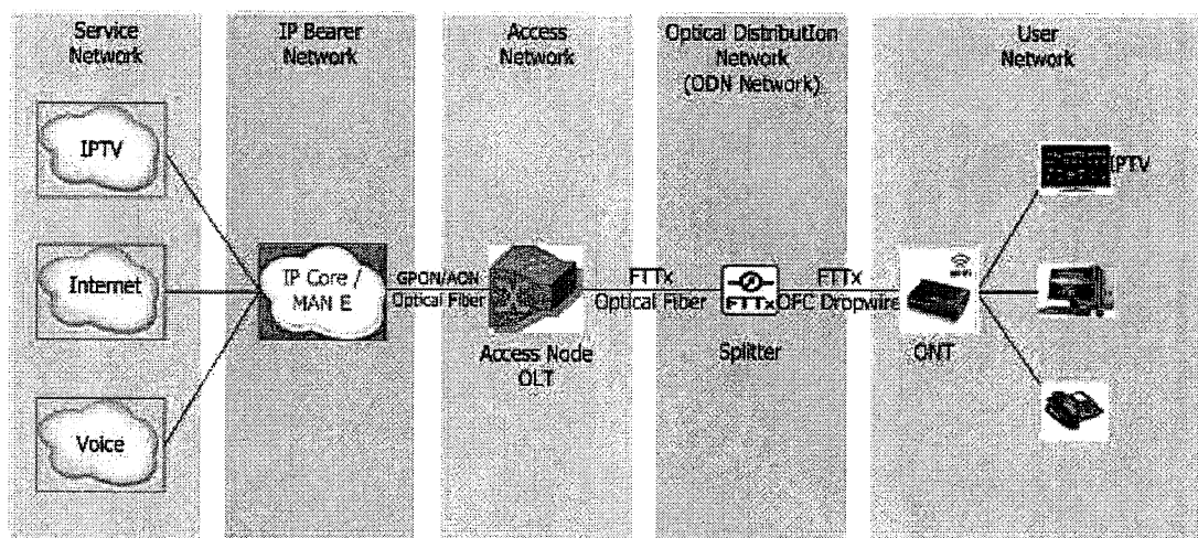
รูปที่ 1 FTTx Network Diagram
