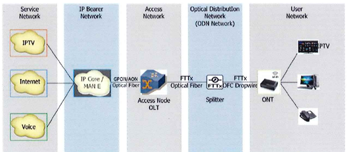
รูปที่ 1 FTTH Network Diagram
